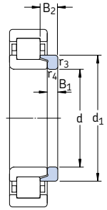
Anelli reggispinta
