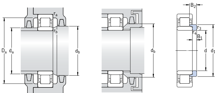
Anelli reggispinta
