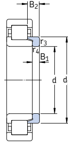
Anelli reggispinta
