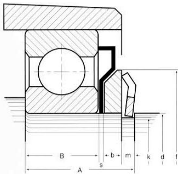
NILOS-Distanzring Typ A mit NILOS-Ring AV (außen dichtend) NILOS-Spacer-Ring type A with NILOS-Ring AV (externally-sealing)
